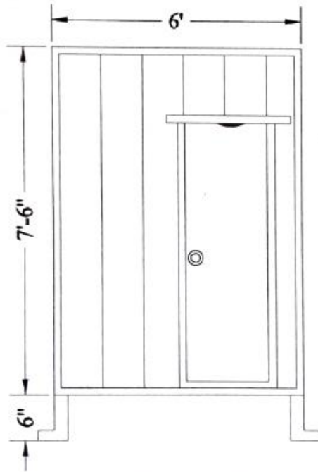
6'X4'X8' Toilet Porta cabin
